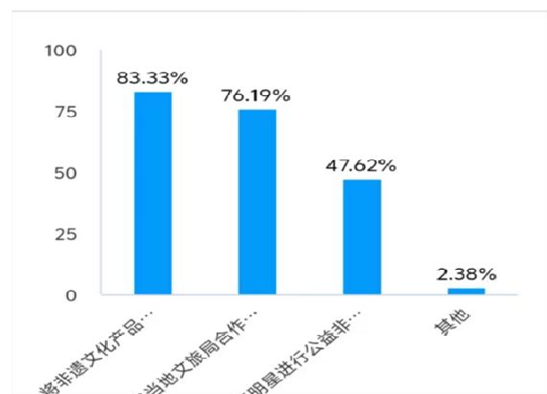
图1 调查问卷
